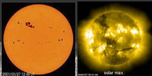
太陽の黒点活動 と乱流渦
